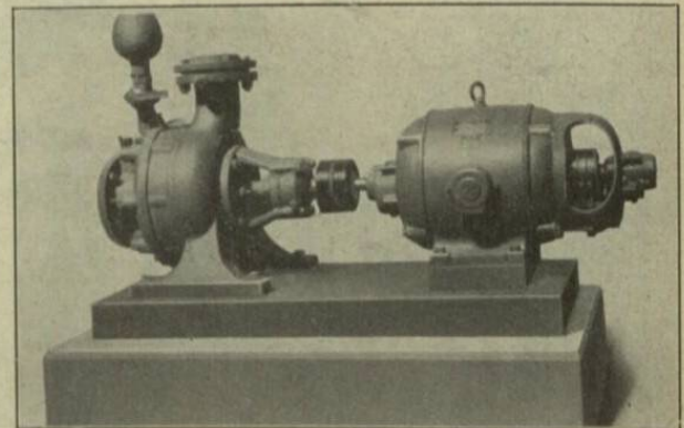
Nahoře stabilní elektrická čerpací souprava pro větší závlahové objekty. — Dole Rot Revolt 3 N v činnosti.
